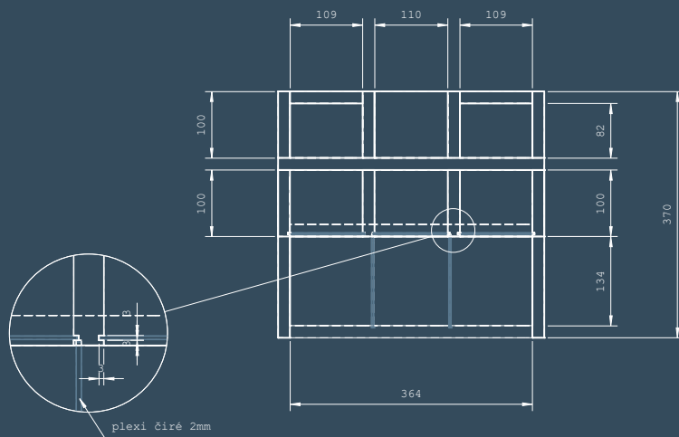
Půdorys M (1:10)
