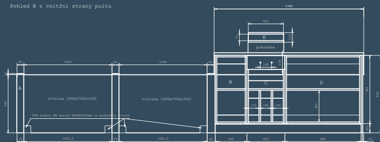
Nárys
