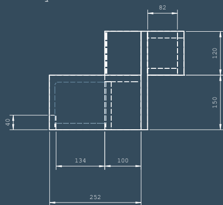
Půdorys M (1:10)
