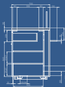
REZ B-B
