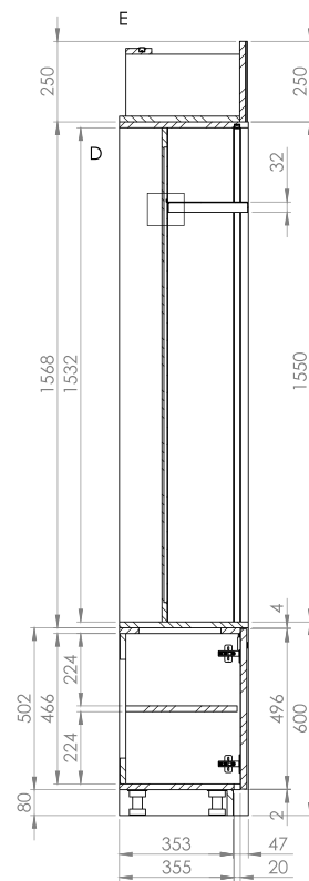
ŘEZ A-A
