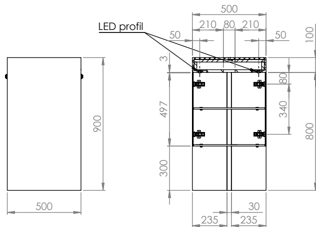
ŘEZ A-A
