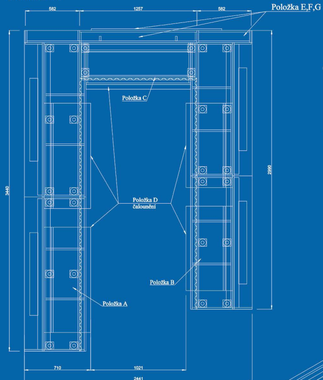
Celková sestava
