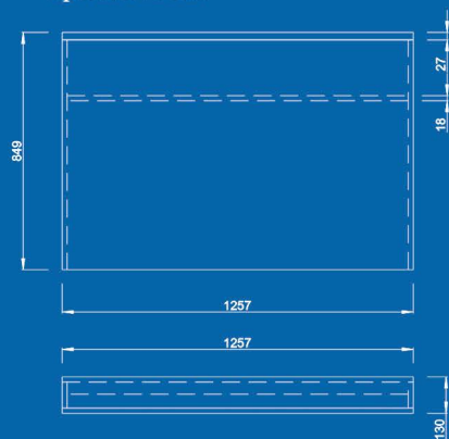
Opěradlová část
