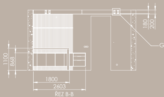
ŘEZ B-B
