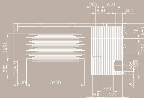
ŘEZ A-A
